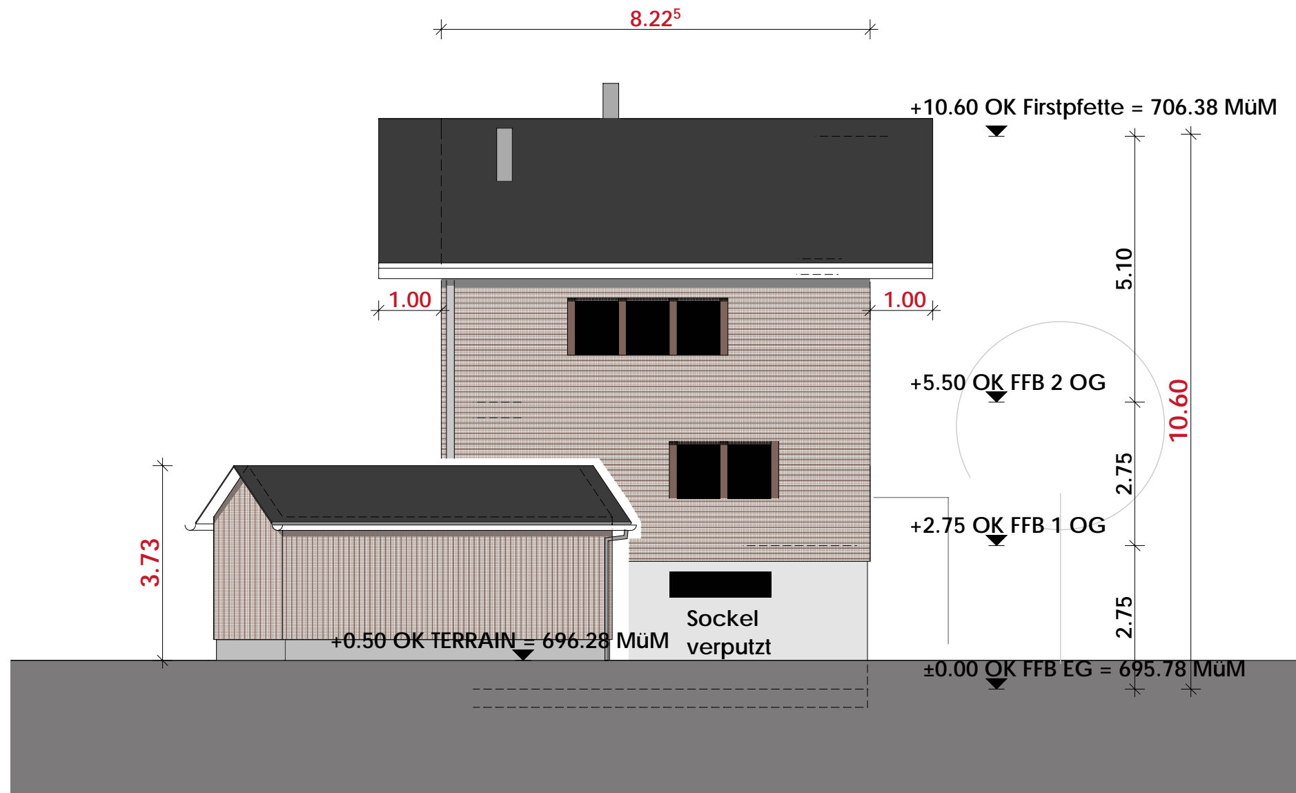
Ansicht Süd West
