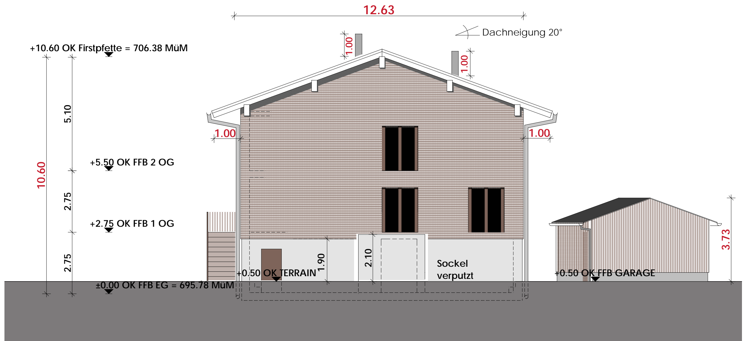
Ansicht Nord West
