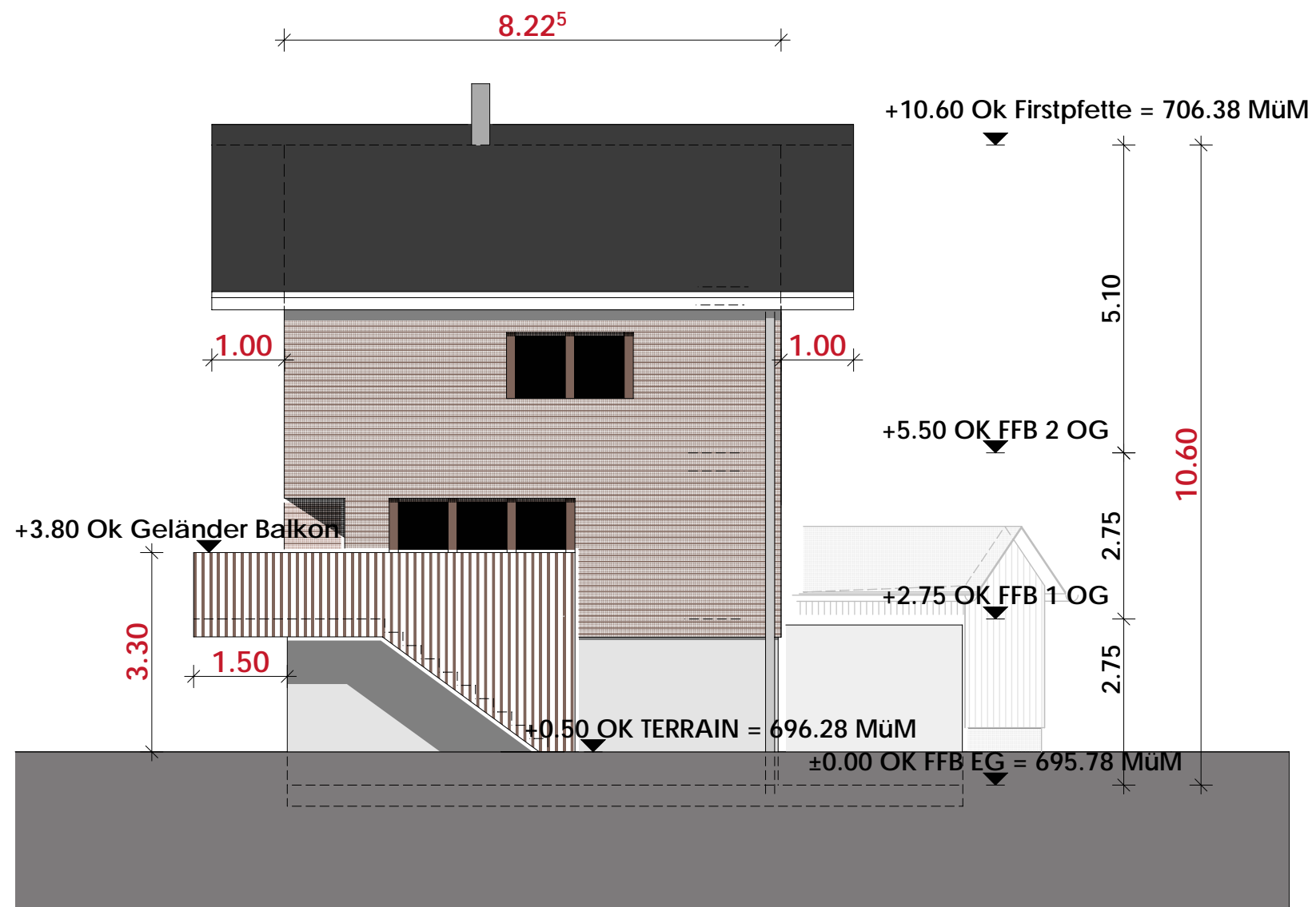
Ansicht Nord Ost
